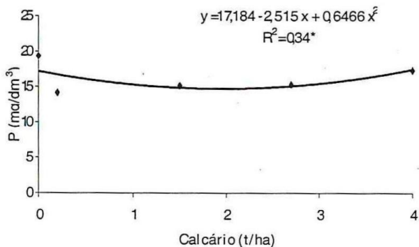
Figura 3 – Efeito da calagem sobre a concentração de fósforo em substrato de Latossolo Amarelo na camada de 0 cm a 30 cm.
