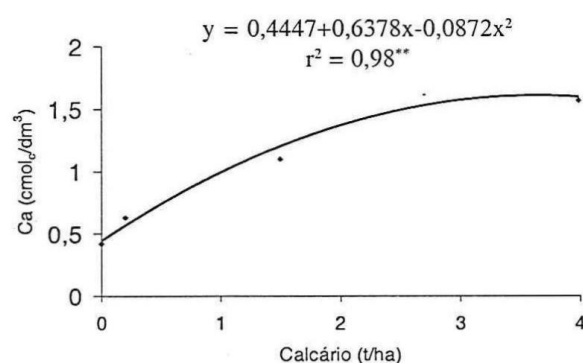
Figura 2 – Efeito da calagem sobre a concentração de cálcio em substrato de Latossolo Amarelo na camada de 0 cm a 30 cm.
